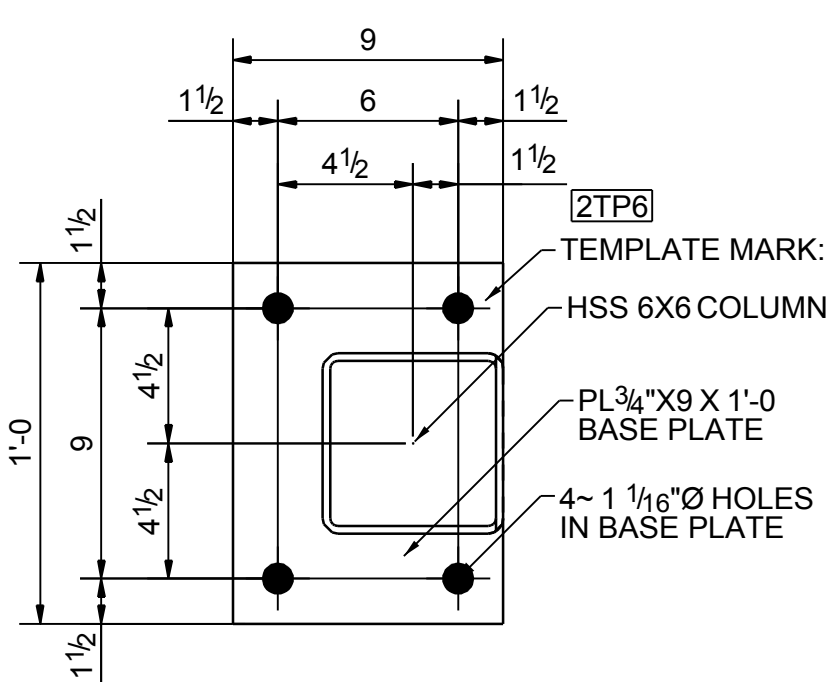
TYPE-8
