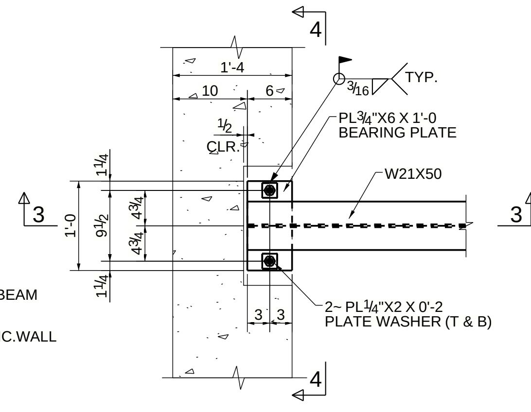
TYPE-8
