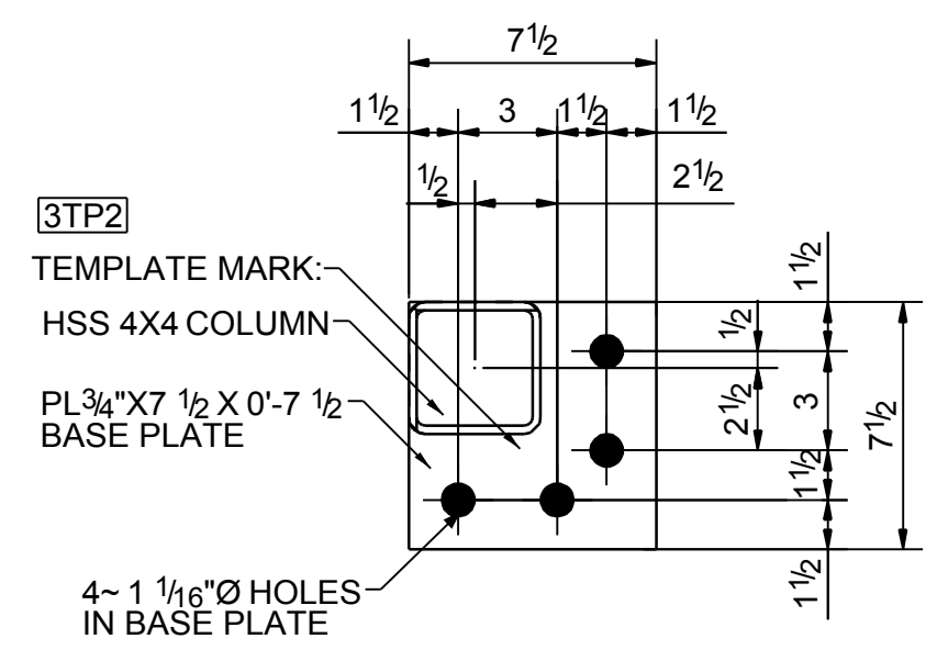
TYPE-11
