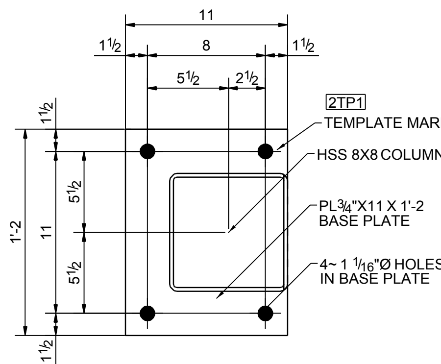
TYPE-9
