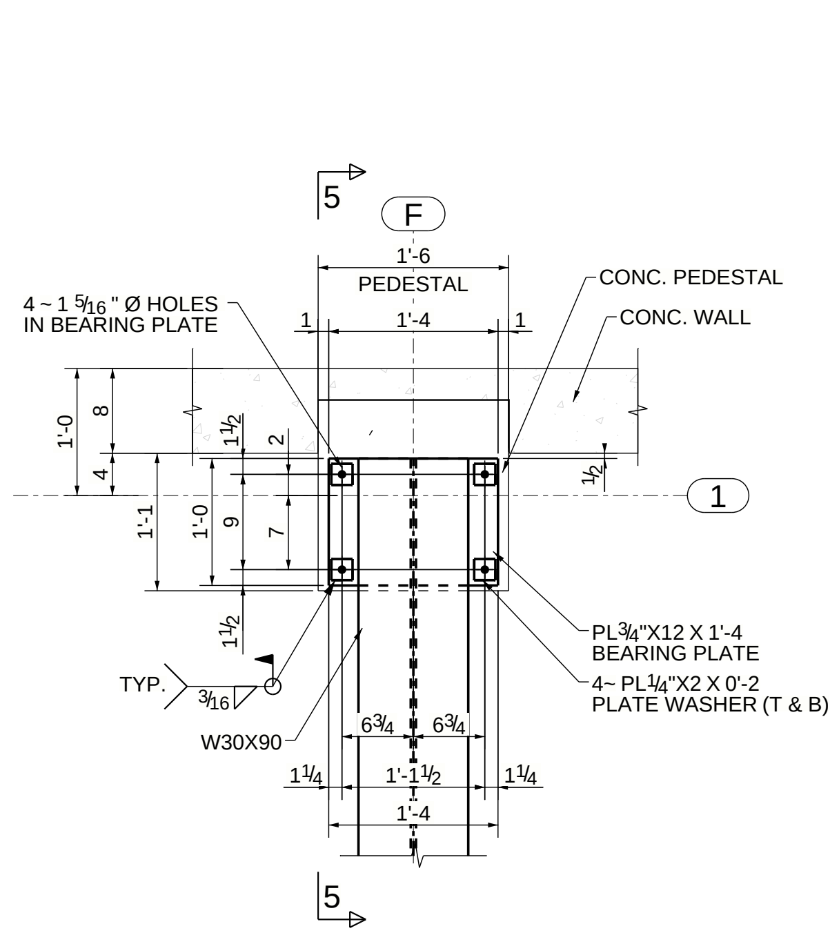
TYPE-9
