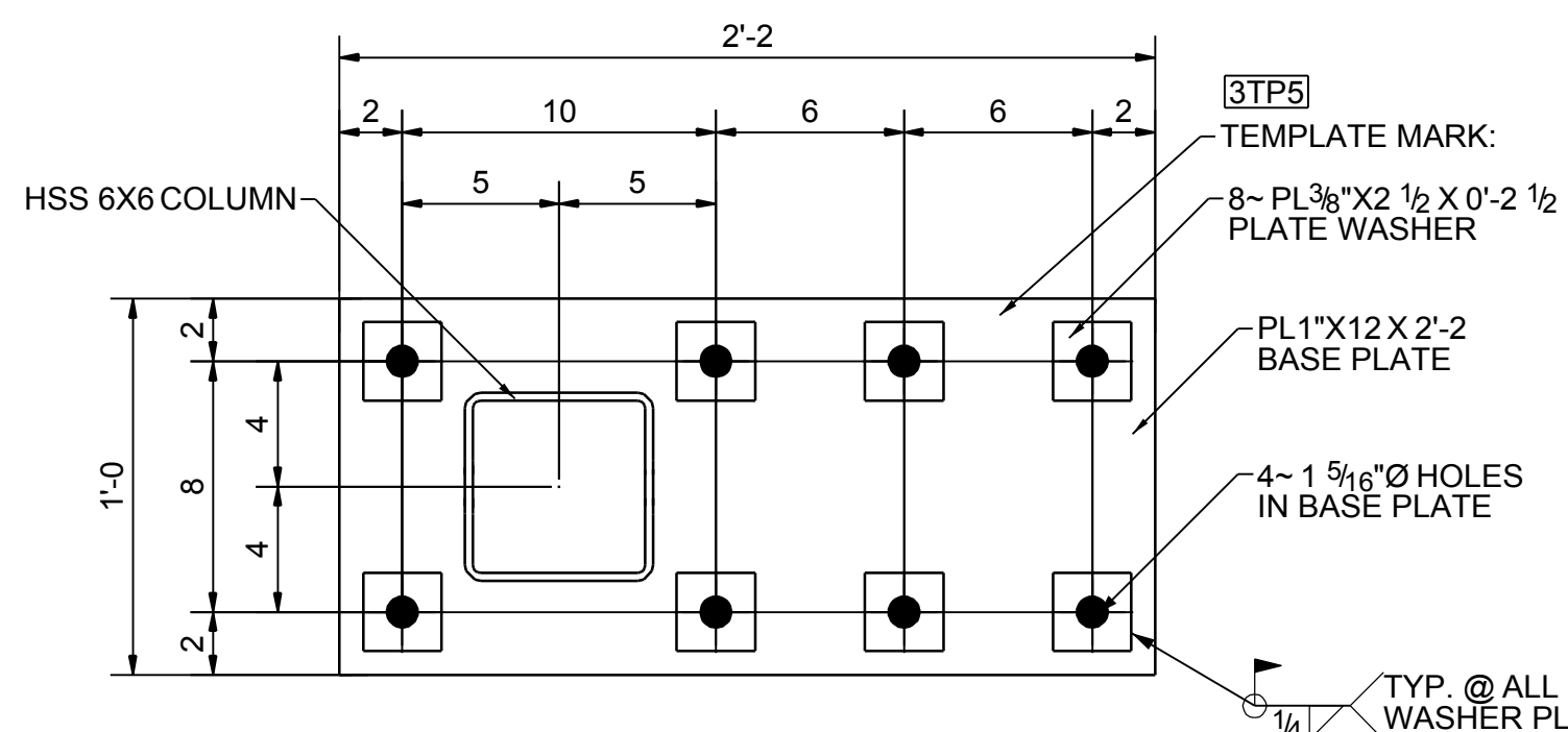
TYPE-14
