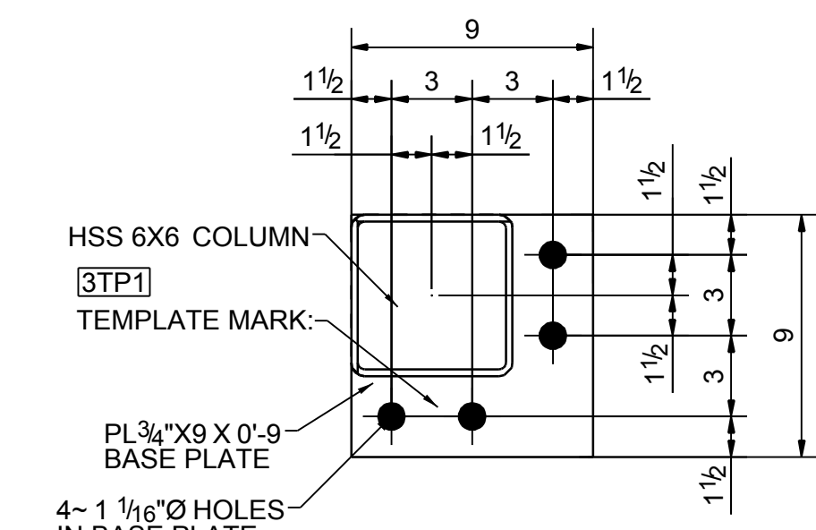
TYPE-12
